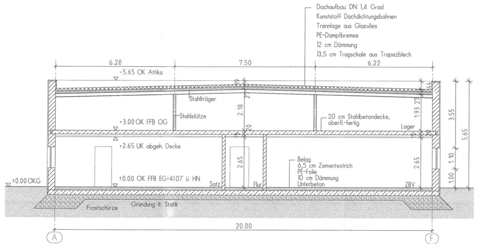
Schnitt B-B
