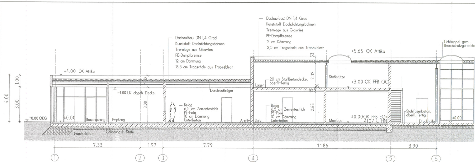
Schnitt A-A
